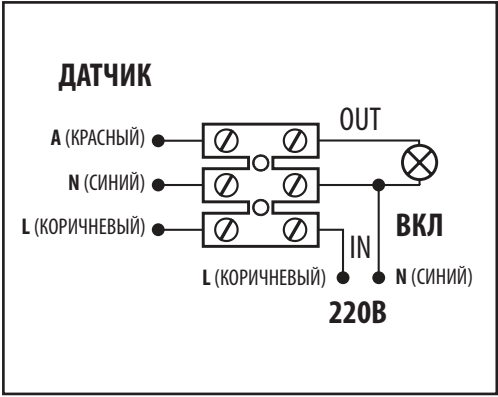
Рис 1. Схема подключения датчика
